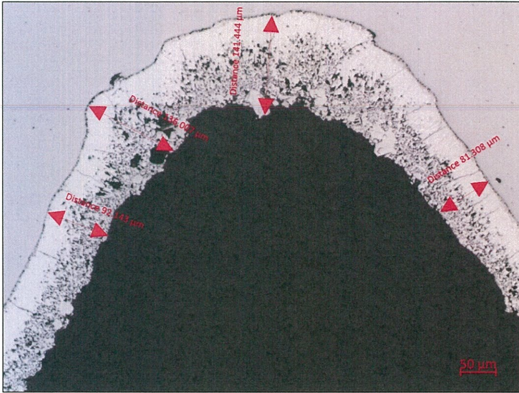
איור 2- תמונת חתך מטלוגרפי אורכי של עוגן החץ
