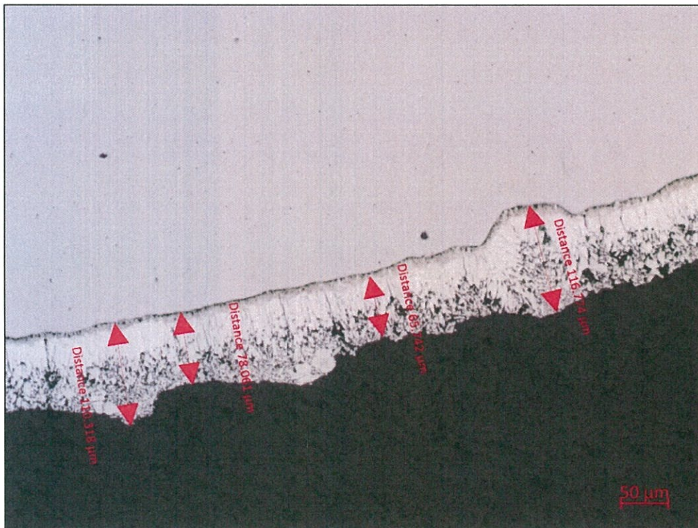
איור 3- תמונת חתך מטלוגרפי רוחבי של עוגן החץ
